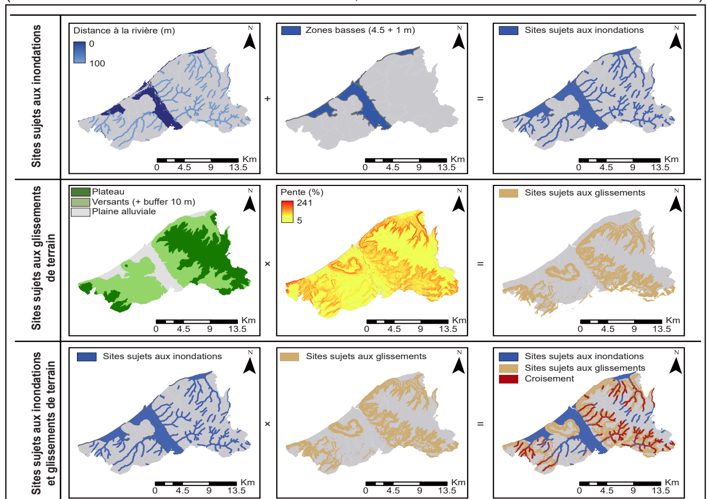
Figure 5 : Détermination des trois types de secteurs potentiellement sujets aux inondations, aux glissements de terrain et aux deux phénomènes (Graff, 2020)
