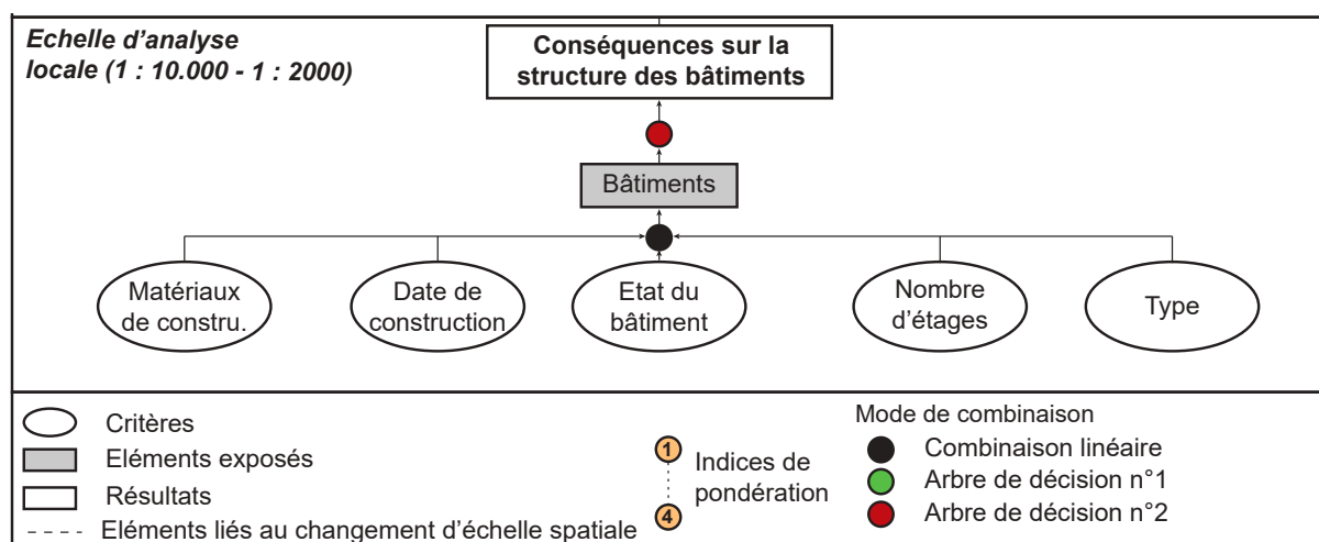
Figure 4 : Organisation du modèle de quantification APC (Affectation, Pondération et Combinaison) à l'échelle locale (Graff, 2020)
