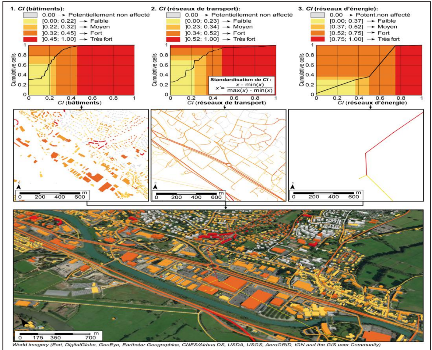
Figure 7 : Calcul des conséquences infrastructurelles (CI) à une échelle large (1 : 25 000 – 1 : 10 000) réajusté en fonction du système de pondération (Dt1). Illustration sur une vignette calée de part et d'autre de la vallée de la Touques du territoire n°1 (Graff et al. , 2019)
