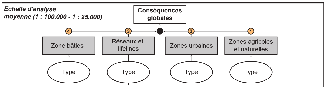
Figure 2 : Organisation du modèle de quantification APC (Affectation, Pondération et Combinaison) à l'échelle moyenne (Graff, 2020)
