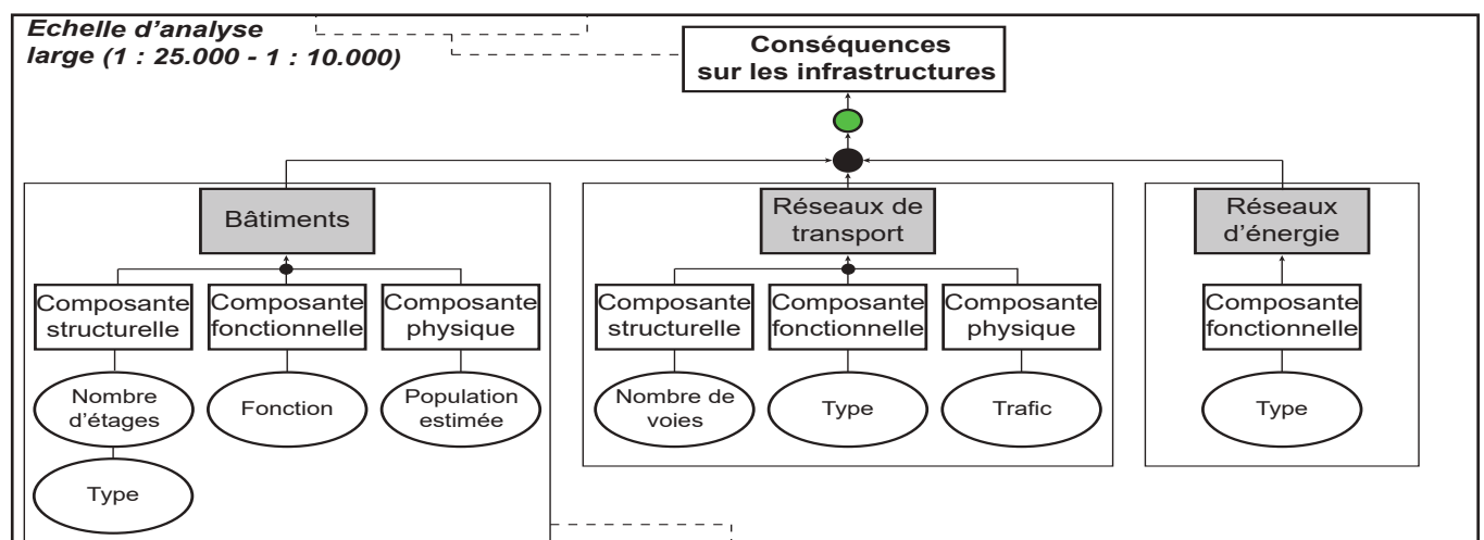
Figure 3 : Organisation du modèle de quantification APC (Affectation, Pondération et Combinaison) à l'échelle large (Graff, 2020)
